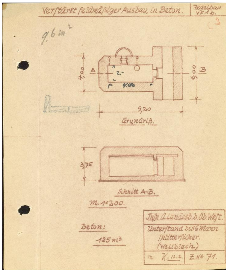
▲ Het standaard bouwwerk dat als basis heeft gediend voor de schuilplaats. Een Vf1b Unterstand bis 6 Mann splittericher (Wellblech). Bron: NIMH 575, 176
