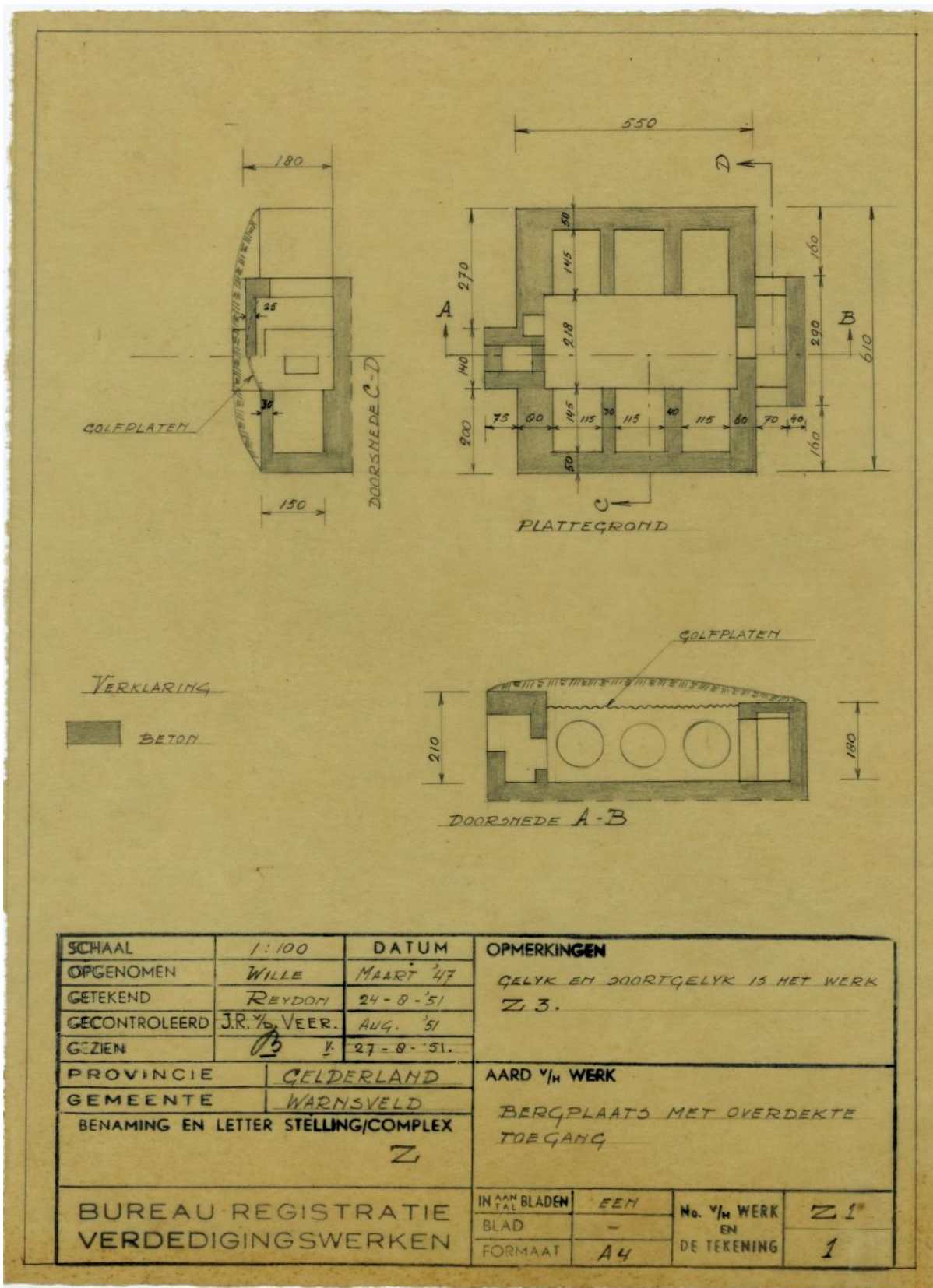
▲ De registratietekening die in 1951 is getekend door het Bureau Registratie Verdedigingswerken en van toepassing is op de groepsschuilplaatsen aan de Rhienderinklaan en op het terrein van Huize Baank.
