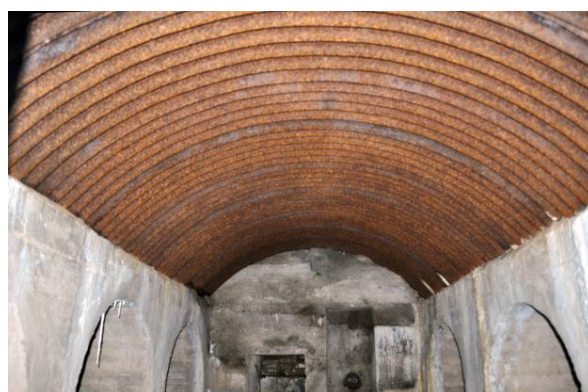
▲ Het interieur van de schuilplaats met het 'Wellblech' dak van het type 'Heinrich'. Foto Leo van Midden 2013
