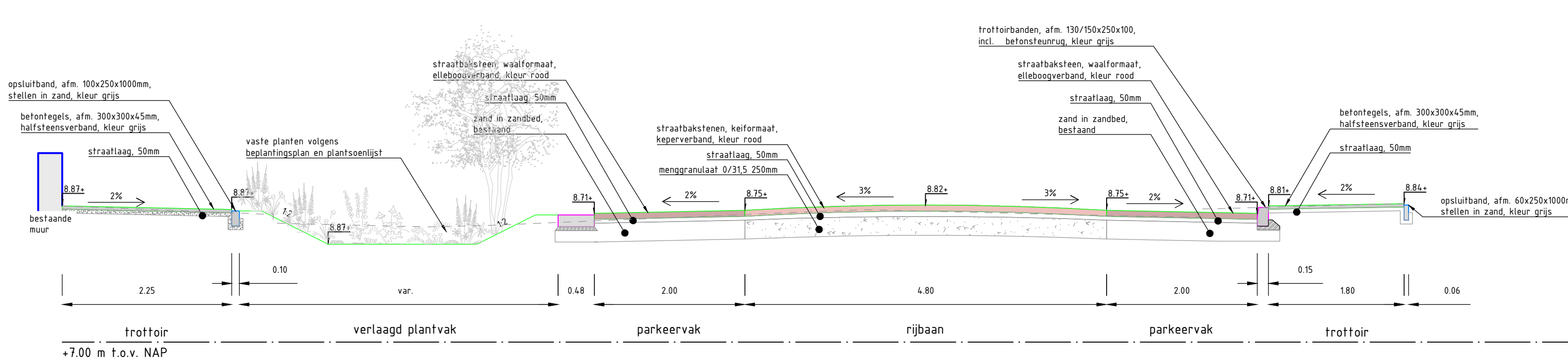
DP03-DP03': principedoorsnede SCHAAL 1:50
