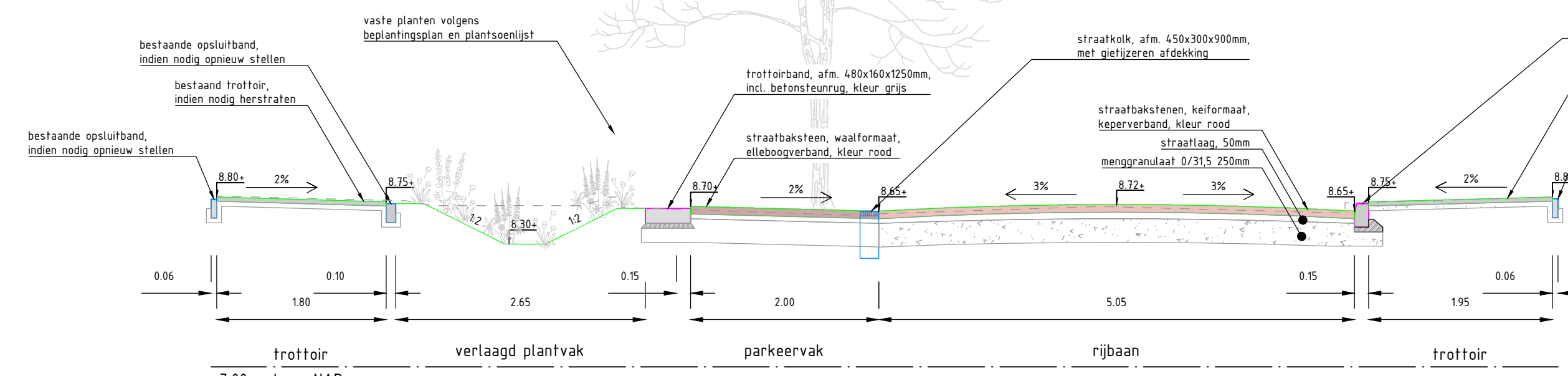
DP01-DP01': principedoorsnede SCHAAL 1:50
