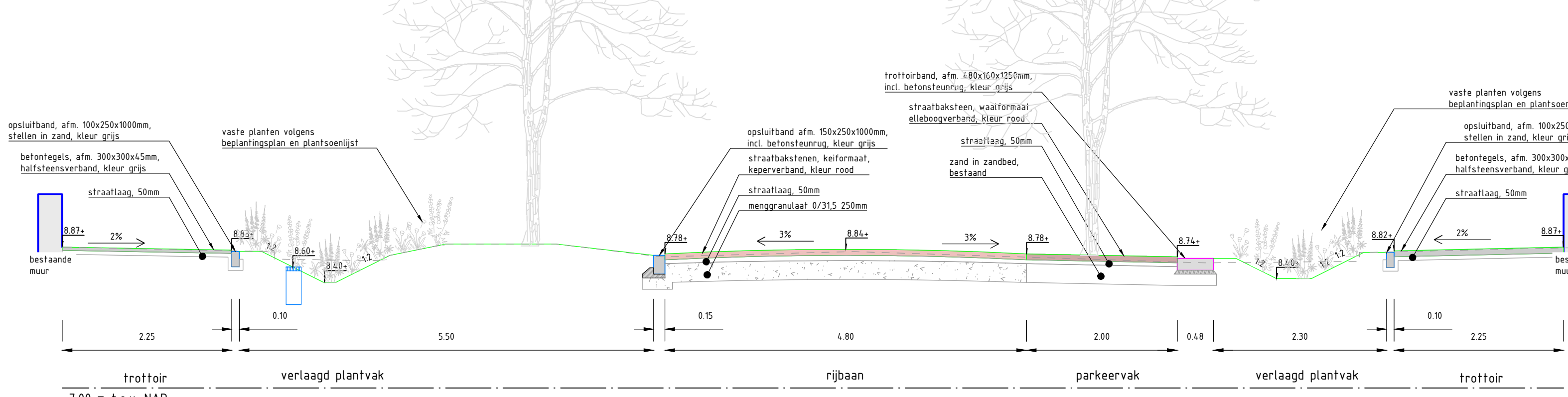
DP04-DP04': principedoorsnede SCHAAL 1:50
